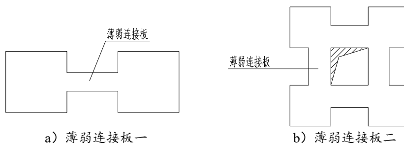
图 1 平面薄弱部位连接板
