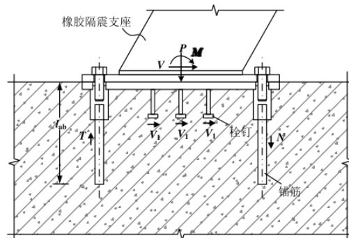
图 D.0.4 预埋件受力情况
