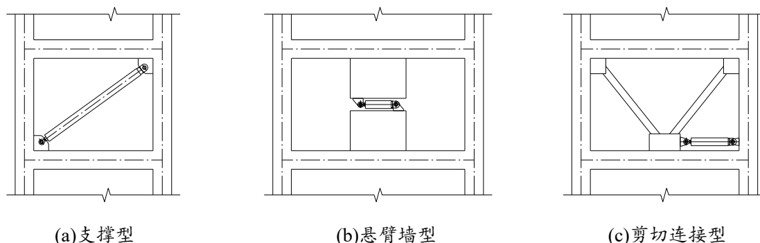
图 5 黏滞消能器消能器常见布置型式
