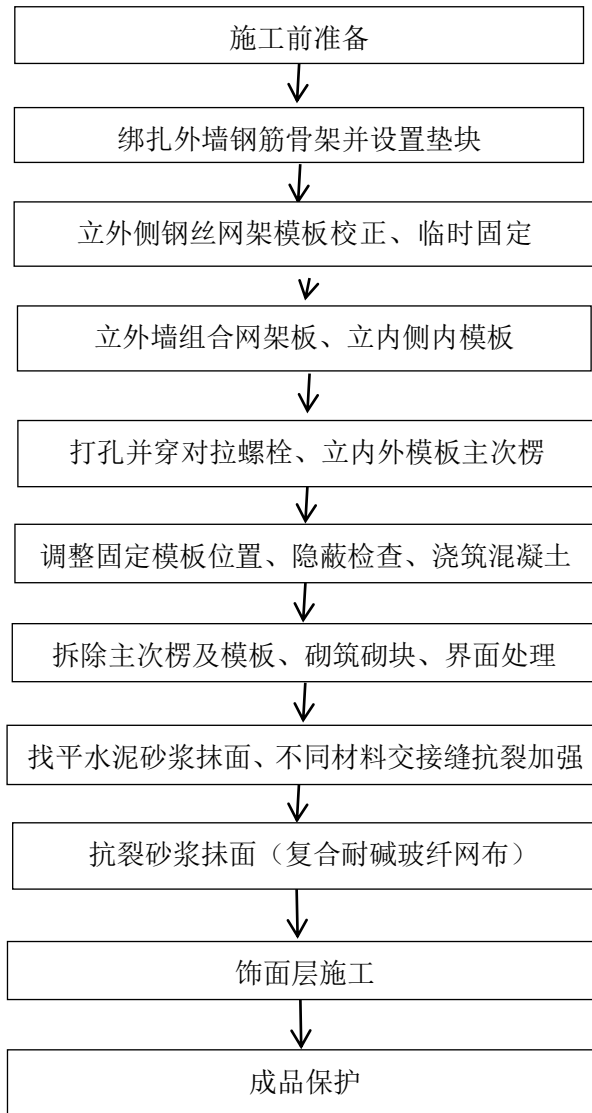
图 6.3.1 钢丝网架免拆模板保温系统施工工艺流程图
