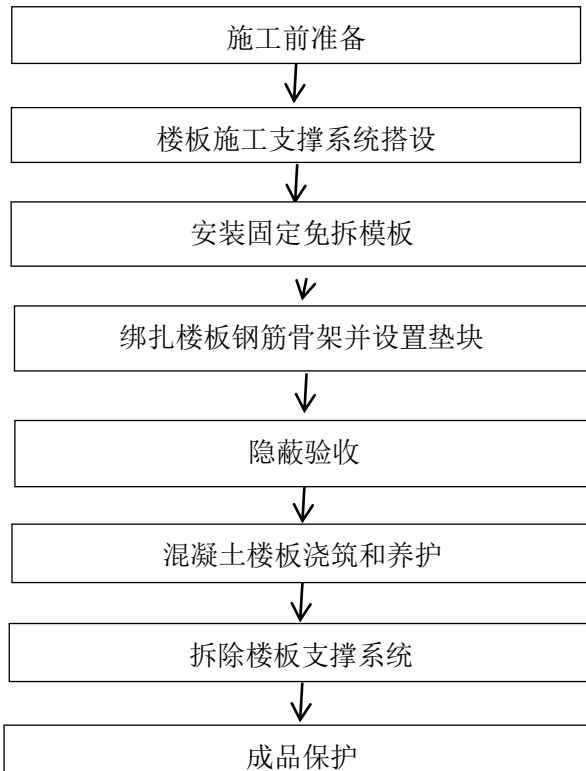
图 6.3.2 钢丝网架免拆模板现浇混凝土复合保温系统施工工艺流程图
