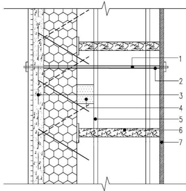
图 6.3.6 轻钢大模框与钢丝网架免拆模板现浇混凝土复合保温系统组装示意图
